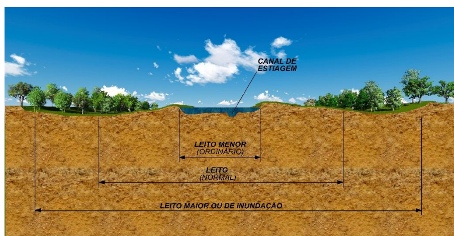
Figura 2: Geomorfologia fluvial
