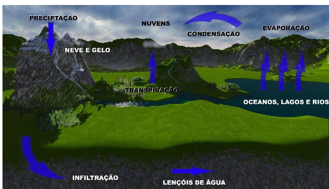
Figura 1: Ciclo Hidrológico
