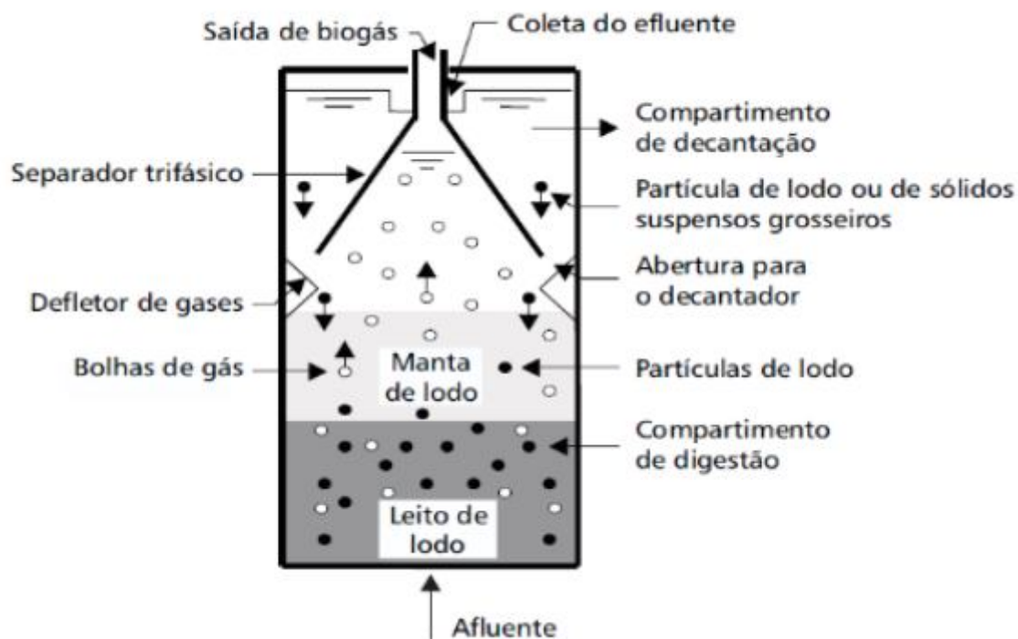
Figura 2: RAFA (Reator Anaeróbico de Fluxo Ascendente). Fonte: Chernicharo et al. 1999
