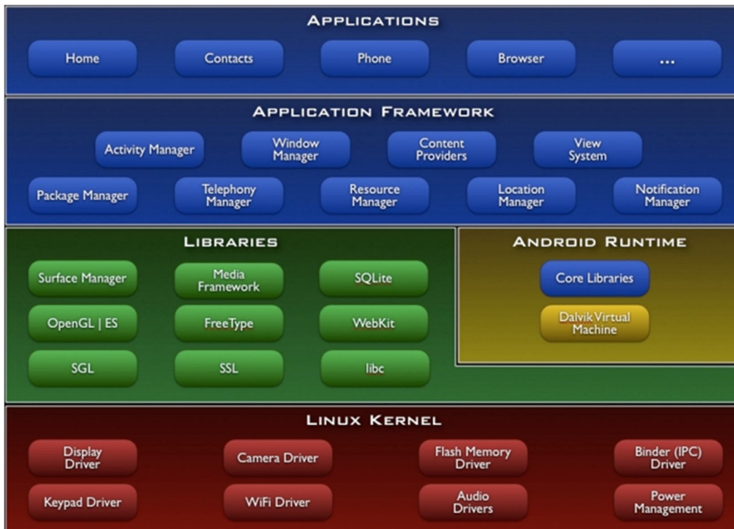
Figura 3: Arquitetura do sistema operacional Android.
