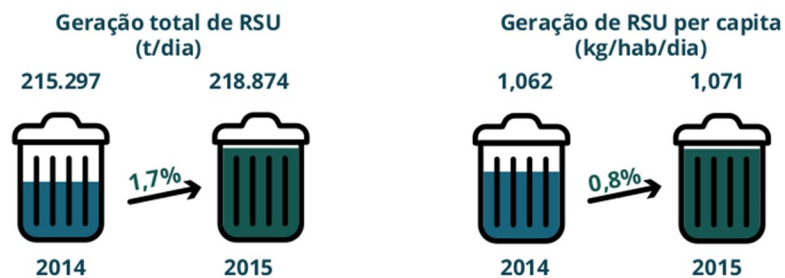
Figura 1: Geração total e per capita de resíduos sólidos urbanos no Brasil.
