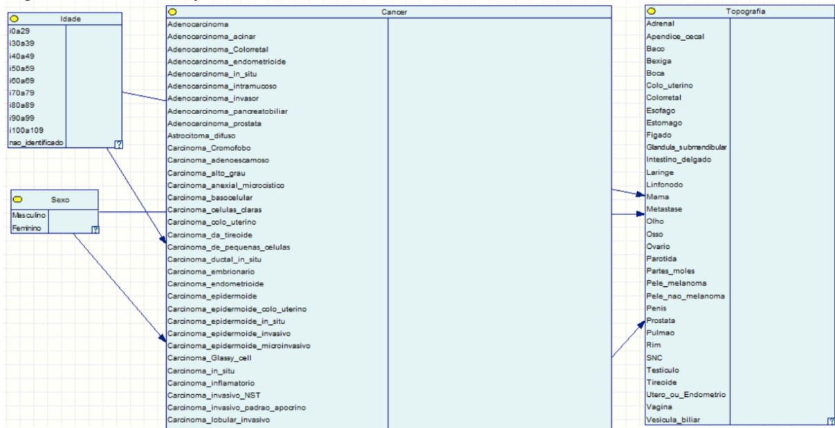
Figura 5 – Rede bayesiana alimentada com os dados
