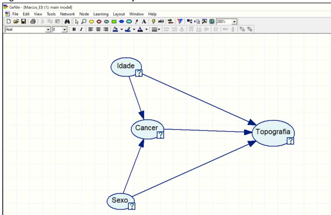
Figura 4 – Estrutura da rede bayesiana
