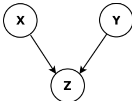
Figura 3 – Grafo modelo de redes bayesianas
